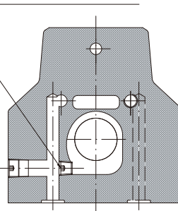
Y-Y 剖面
