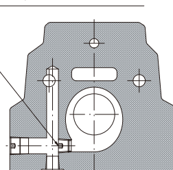
Y-Y 剖面
