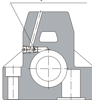
Y-Y 剖面
