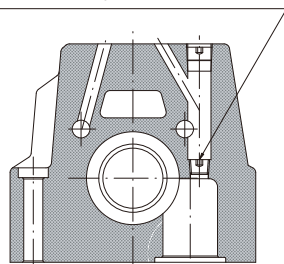
X-X 剖面
