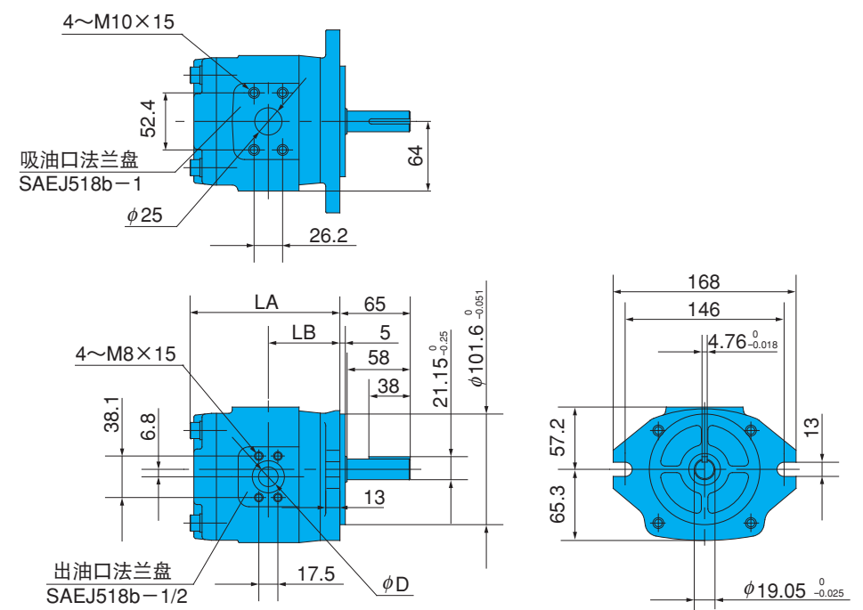
IPH-3B-*-20（法兰式右转）
